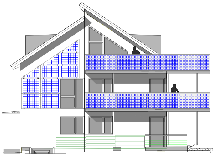
Ansicht Westen
